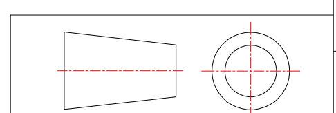
视图A 比例 3:1
